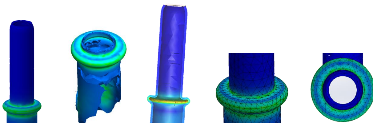
Distribuição da carga uniformemente sobre apoio do tubo
