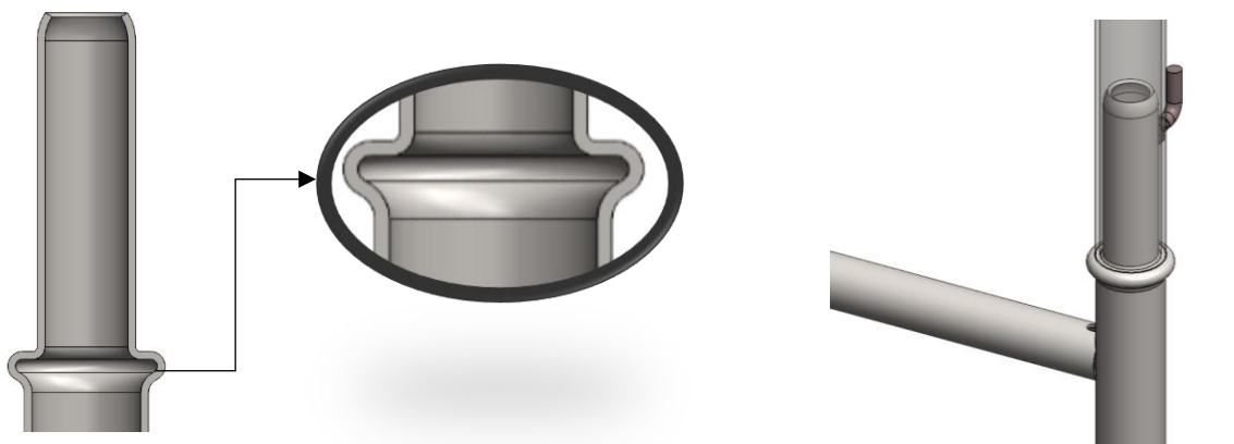
Geometria da ponta e o encaixe interno
